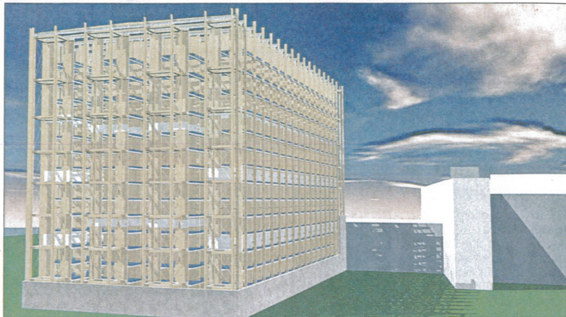
Hochregallager aus 700 m 3 Fichtenholz bei Offsetdruck-Schwarzach.
