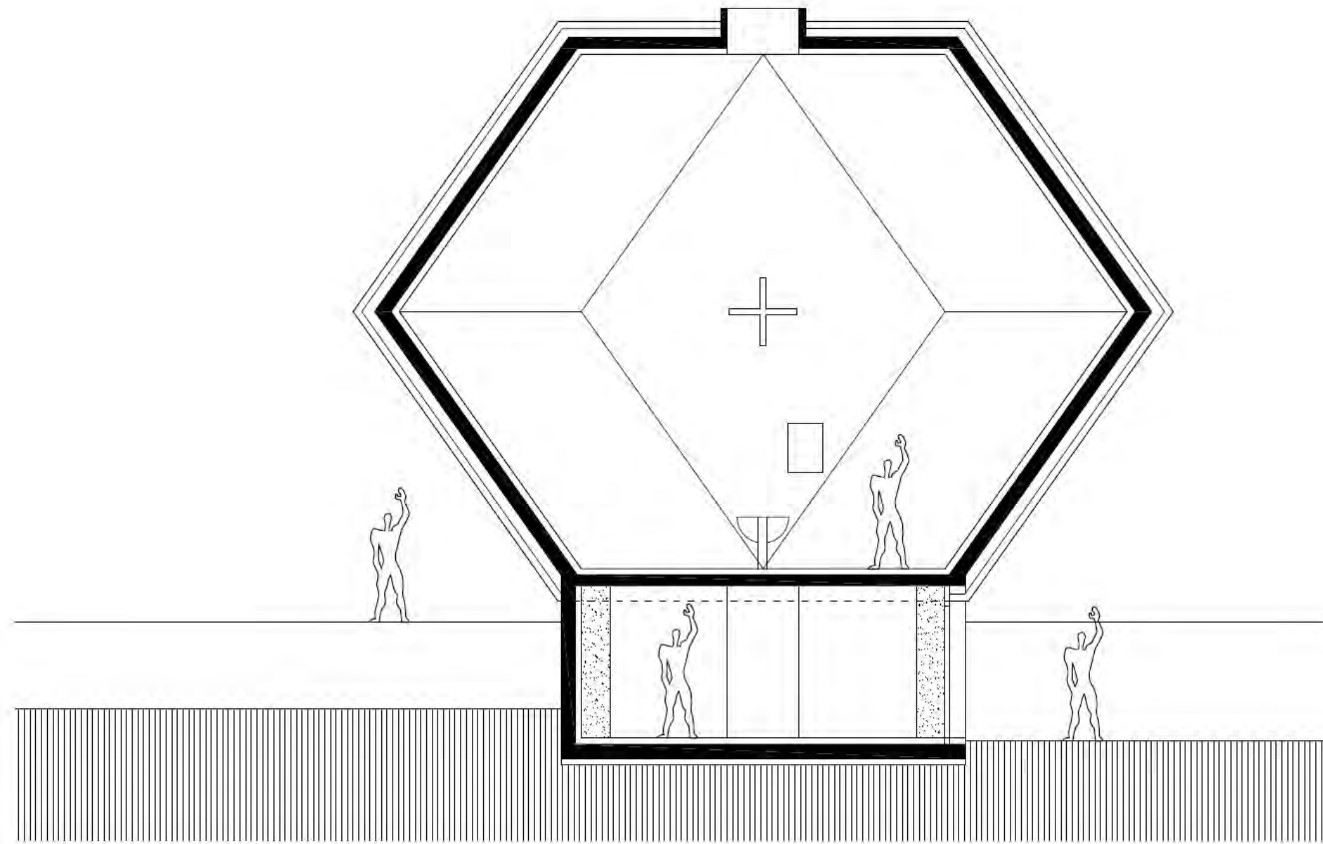
SEZIONE TRASVERSALE/CROSS-SECTION
